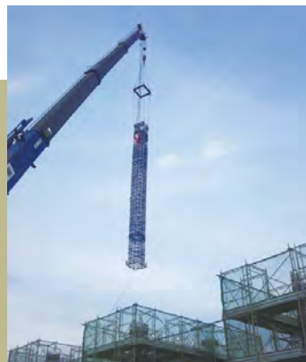
JR平山高架橋[長崎県諫早市]
