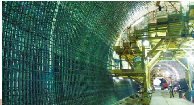
三坂トンネル（組み立て状況）【佐賀県嬉野市】
